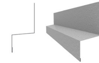
기단부 후레싱
