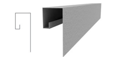
상부 후레싱
